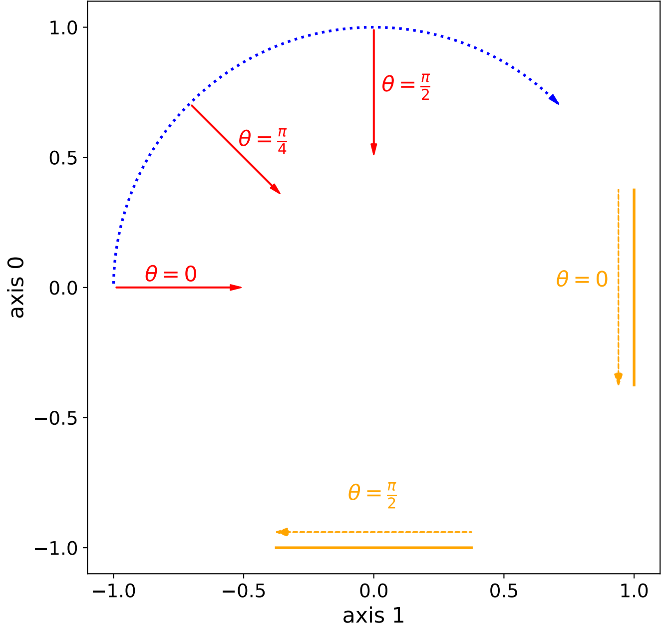
svmbir
