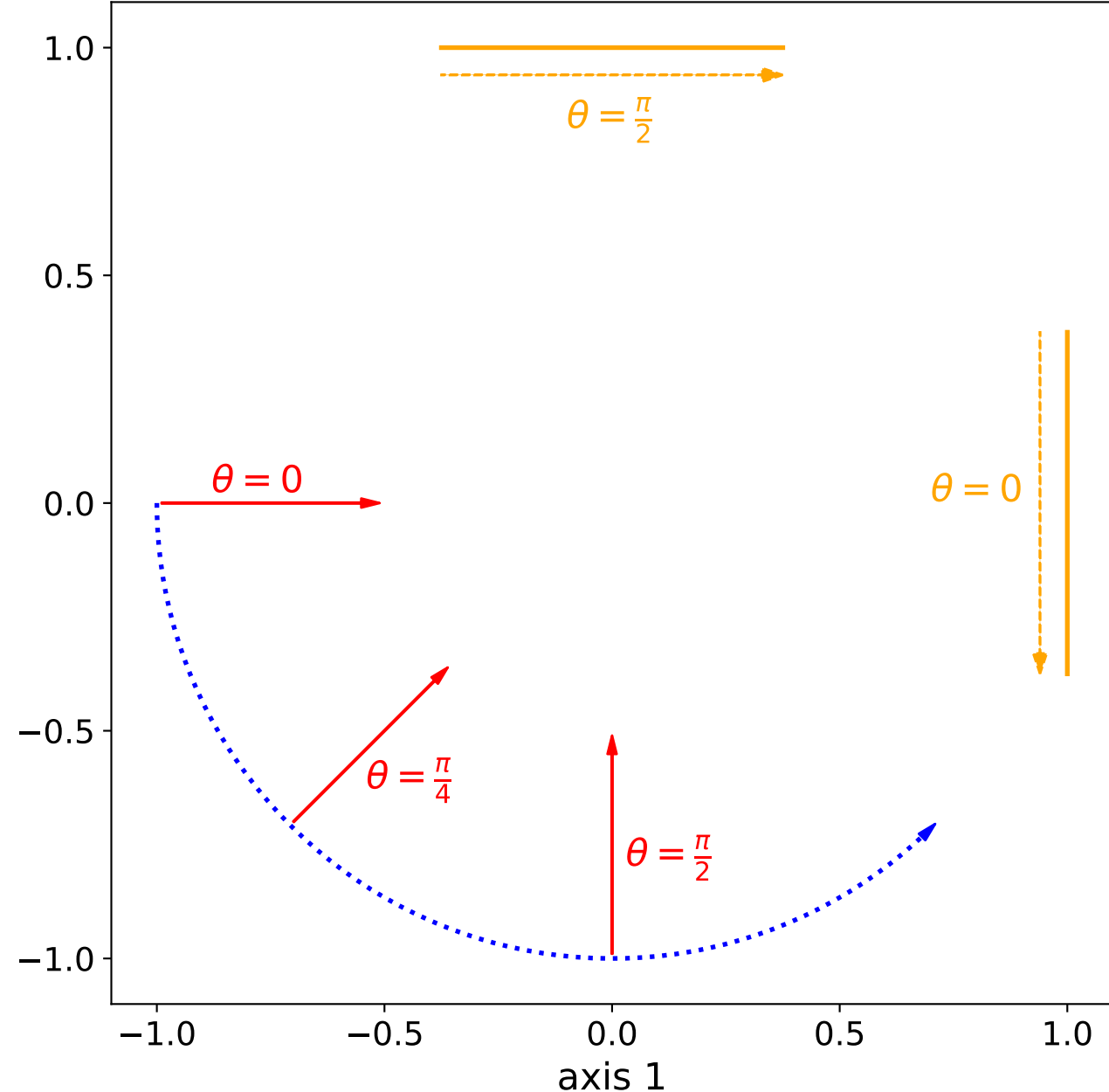
scico
